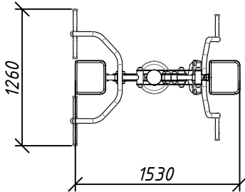
Жим сидячи від грудей – Тяга зверху InterAtletika SL 101.1 М 1:50
