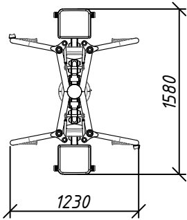
Бамерфляї InterAtletika SL 128 М 1:50
