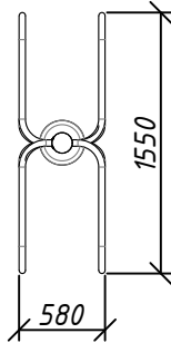
Брусу InterAtletika SL 105 М 1:50
