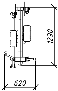
Ордімрек InterAtletika SL 116 М 1:50
